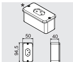
Caixa condutele 5 entradas com tampa e tomada.
