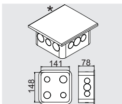
Caixa de passagem elétrica de parede - Embutir.
