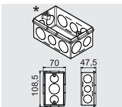
Caixa de Luz - 4"X2"
