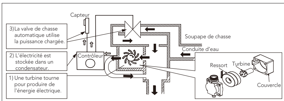
fig. 1 Générateur Hydropowered
