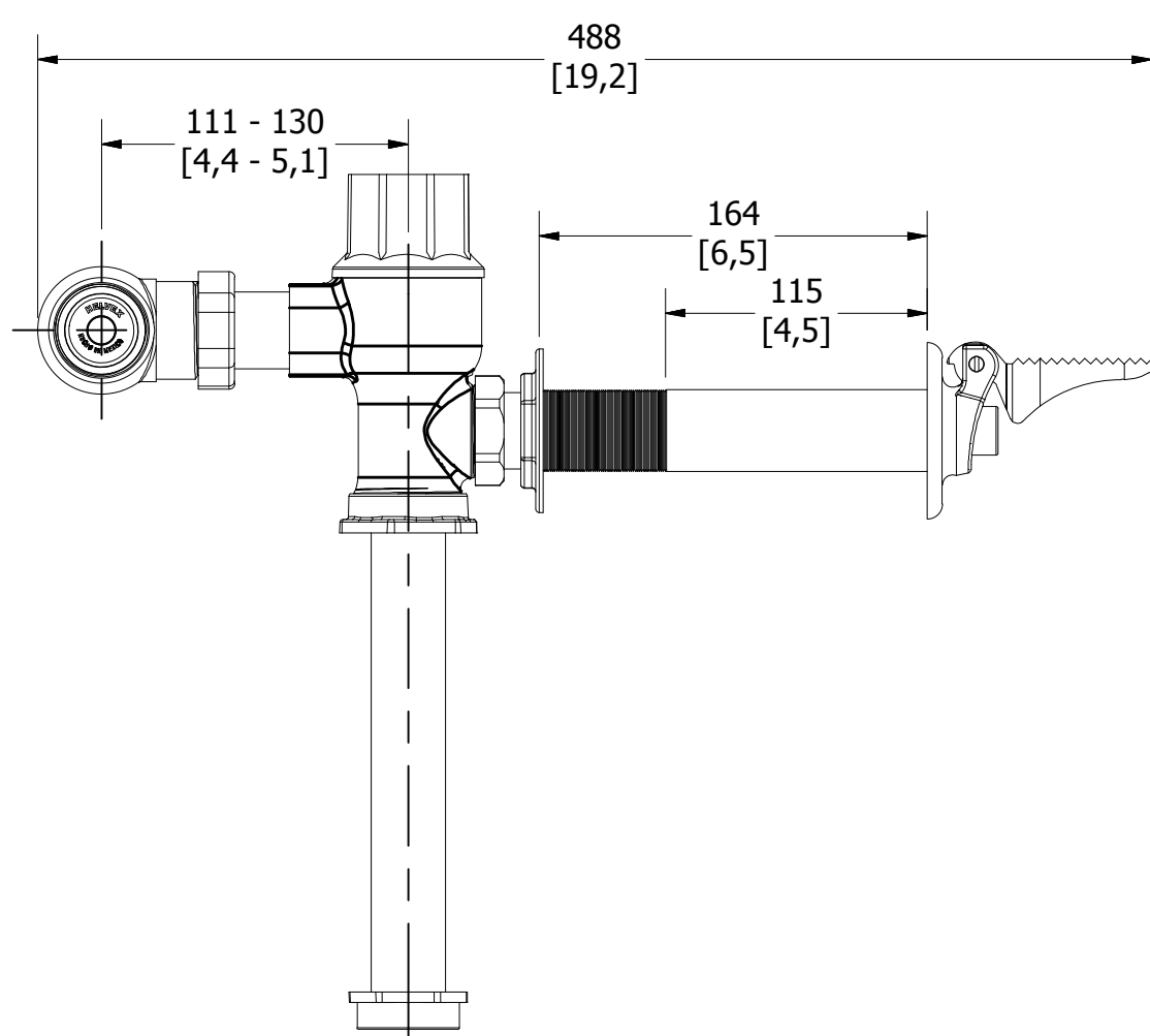
Medidas Referenciales / Estimated Dimensions, Acot.mm.[pulg] / Dim.mm.[in]
