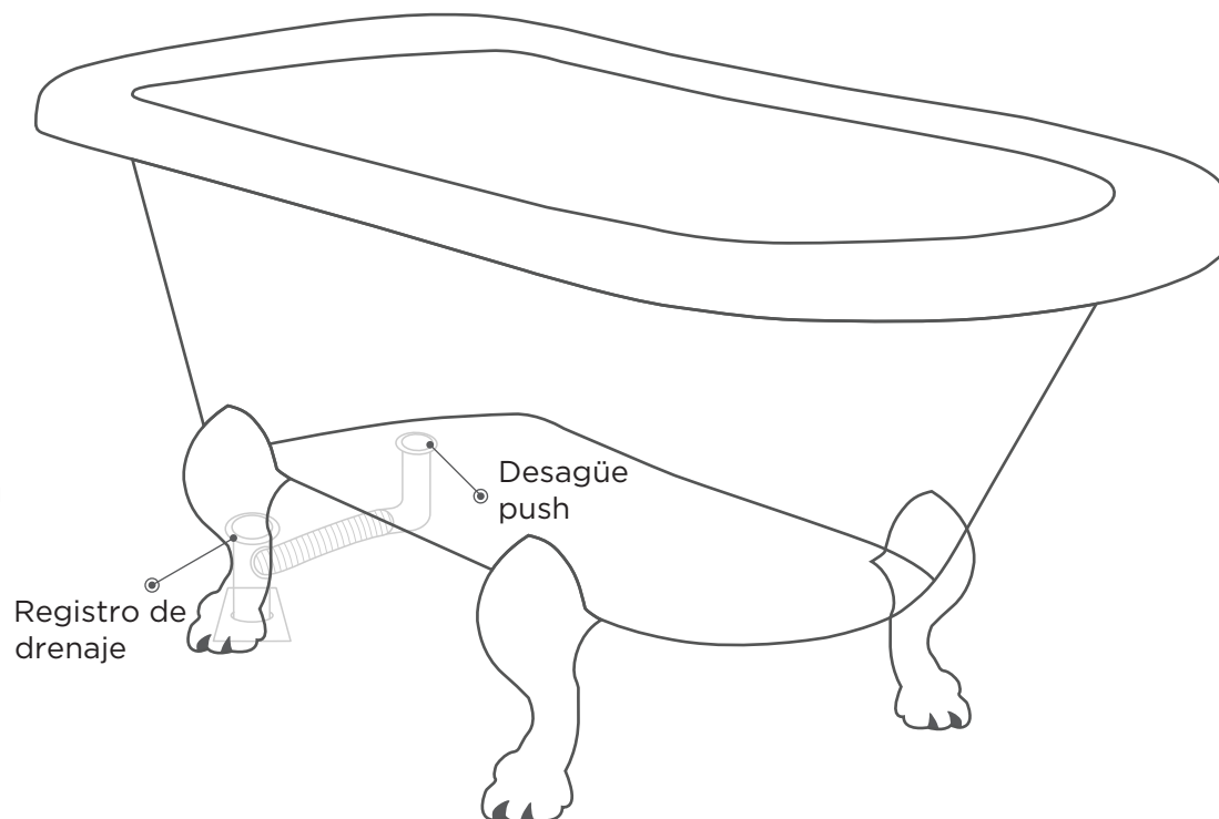
Sistema de llenado por grifo free standing (opcional)
