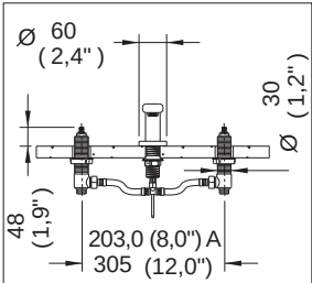
Medidas Referenciales
