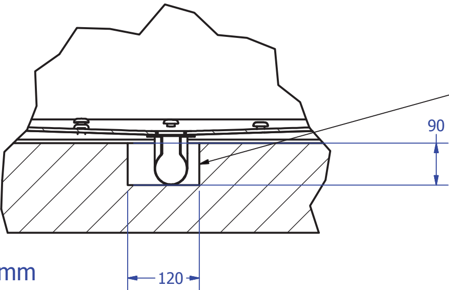
DETAIL B SCALE 0.16 : 1
